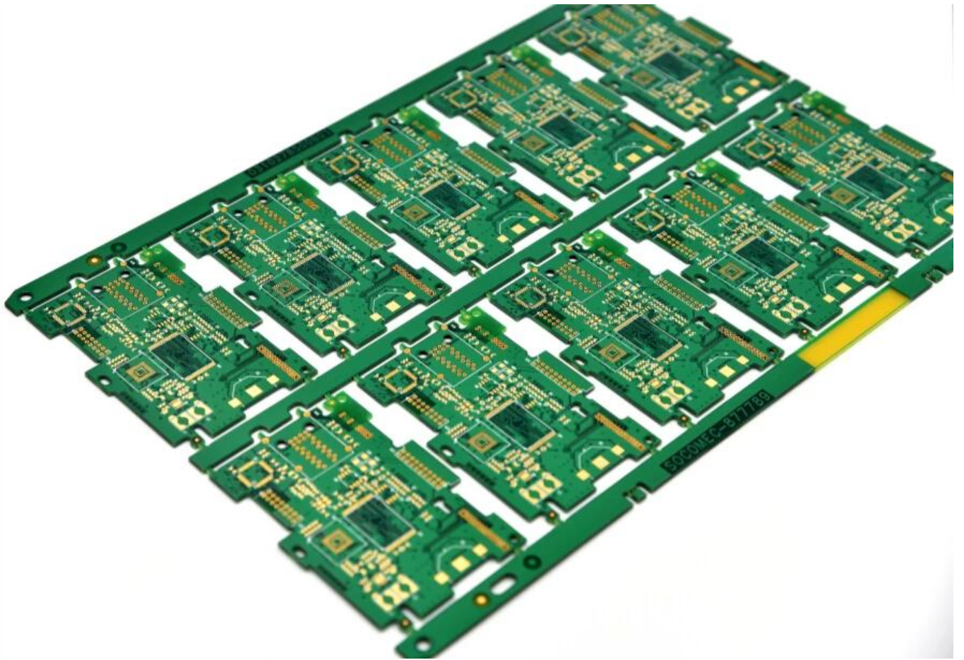
Piiirevyjen valmistus, HDI-piiirevy Printed circuit board, PCB LED-TV; n valmistamiseen
